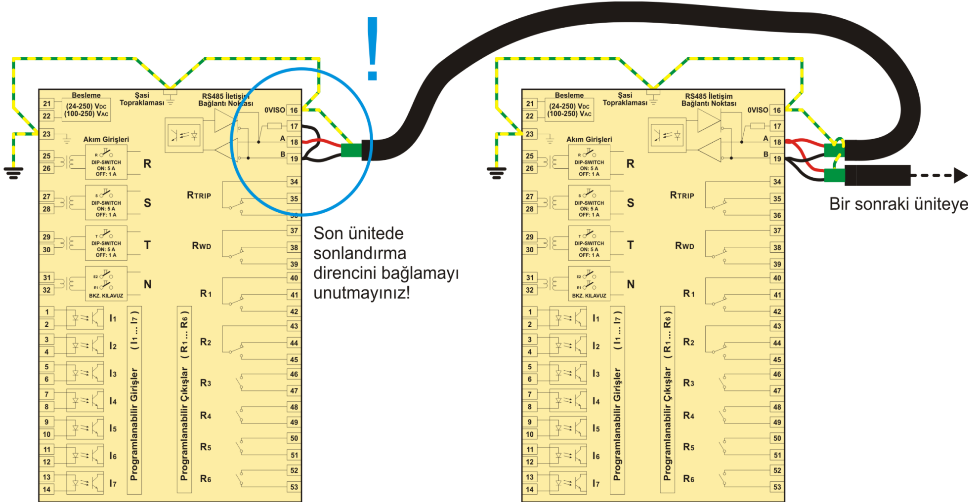
DEMA CPM 310 G Dijital Aşırı Akım Koruma Rölesi RS485 Bağlantı Şeması
